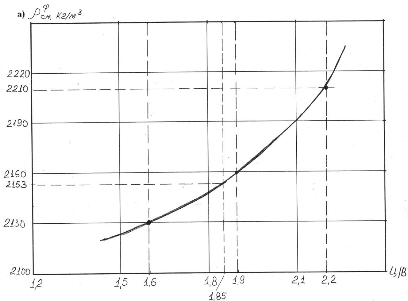
Рисунок 7.1, а – Базовая зависимость: «плотность – Ц/В-отношение»
