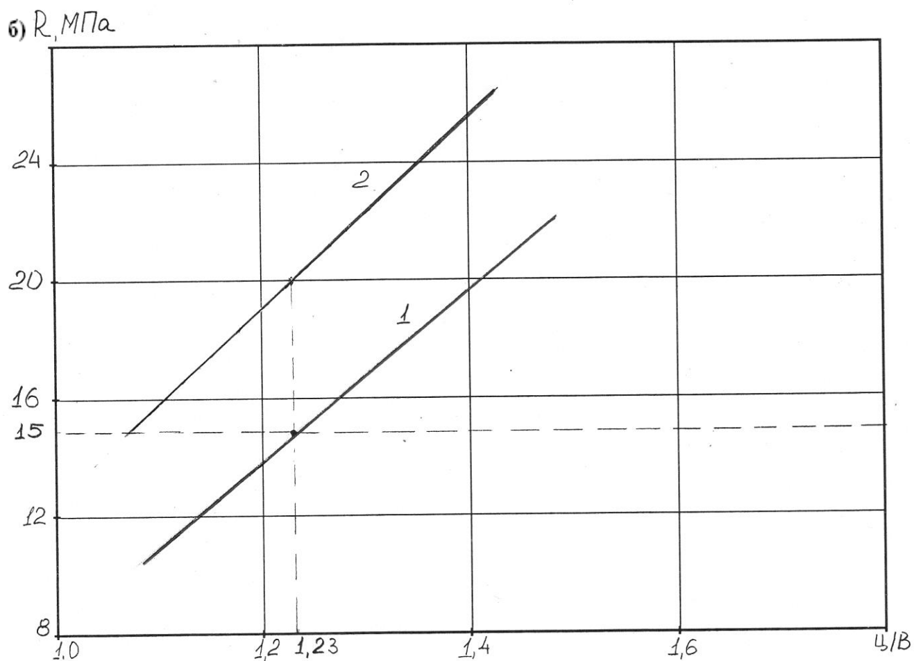
Рисунок 9.3 – Базовая зависимость «прочность – Ц/В-отношение»;
