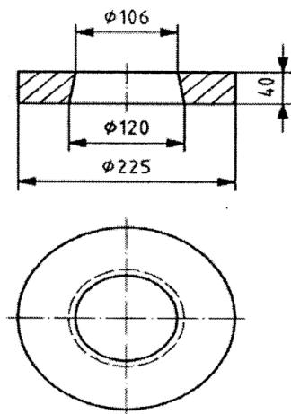
Рисунок 2. Раструб, размеры в мм
