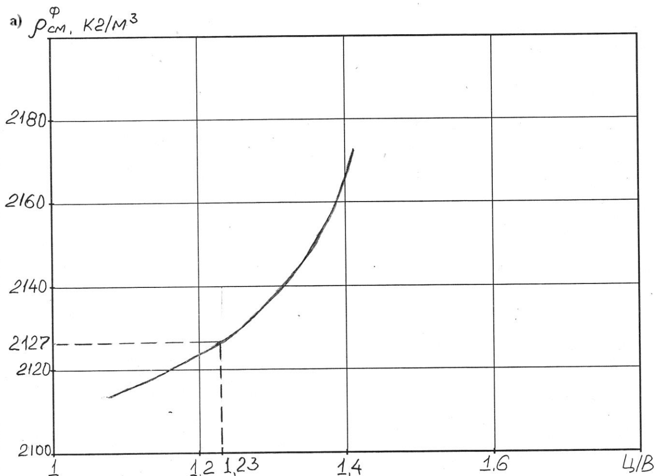
Рисунок 9.2 – Базовая зависимость «средняя плотность бетонной смеси – Ц/В-отношение»
