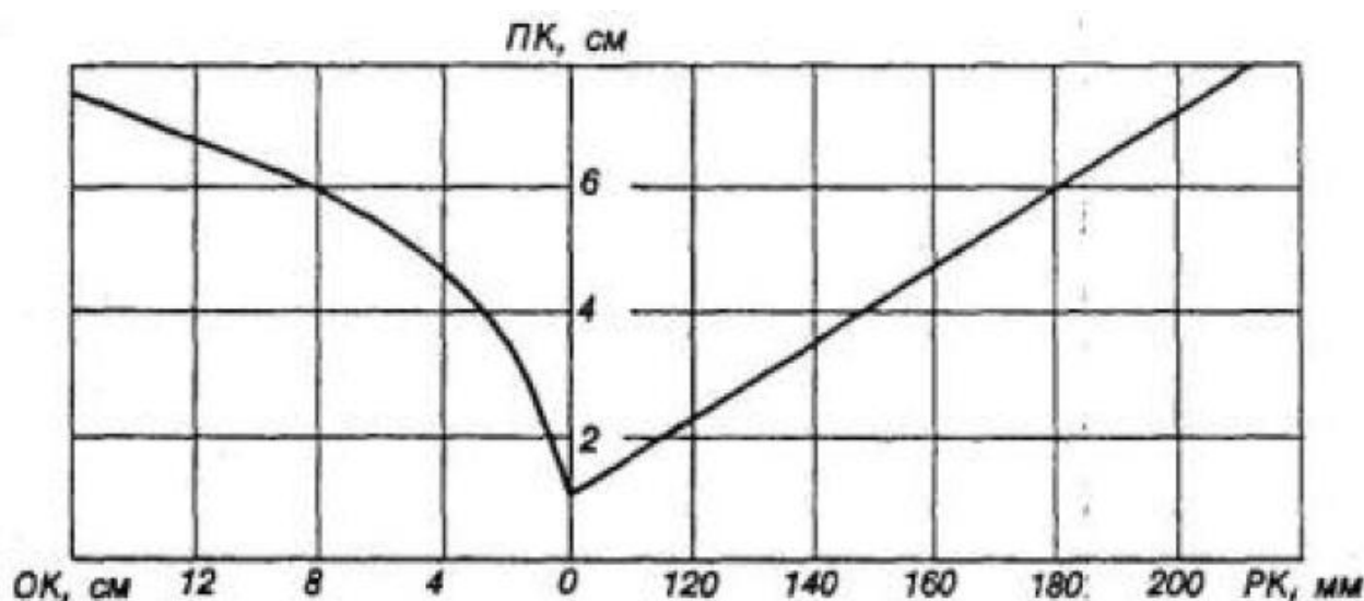
Рисунок 9.1 – Связь показателей осадки конуса ОК, погружения конуса ПК СтройЦНИИЛ и распыла конуса РК на встряхивающем столике для мелкозернистой бетонной смеси
