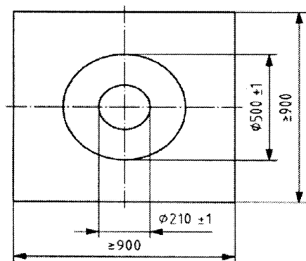
Рисунок 1. Базовая плита, размеры в мм
