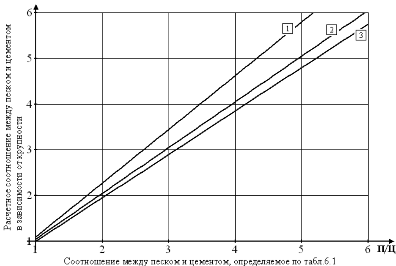
Рисунок 6.2 – Корректирование песко-цементного отношения, обеспечивающего заданную удобоукладываемость; модуль крупности песка: 1 – 3,0; 2 – 2,5; 3 – 2,0.
