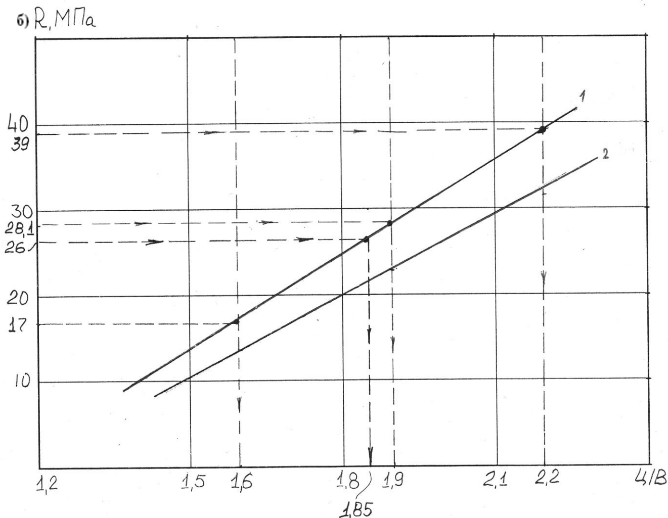
Рисунок 7.1, б – Базовая зависимость: «прочность – Ц/В отношение»; 1 – в возрасте 28 суток; 2 – в возрасте 7 суток
