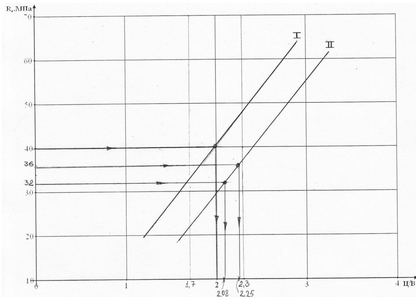
Рисунок 5.2 – Зависимость прочности бетона после тепловой обработки от цементно-водного отношения; I – через 28 суток после тепловой обработки; II – через 4 часа после тепловой обработки
