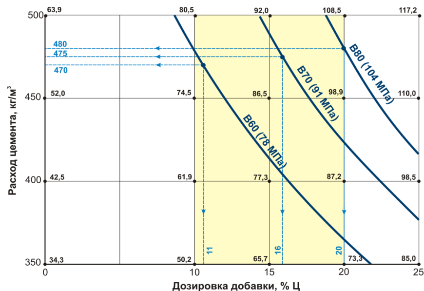
Рисунок 11.2 – Зависимость прочности бетона от расхода цемента и дозировки добавки
