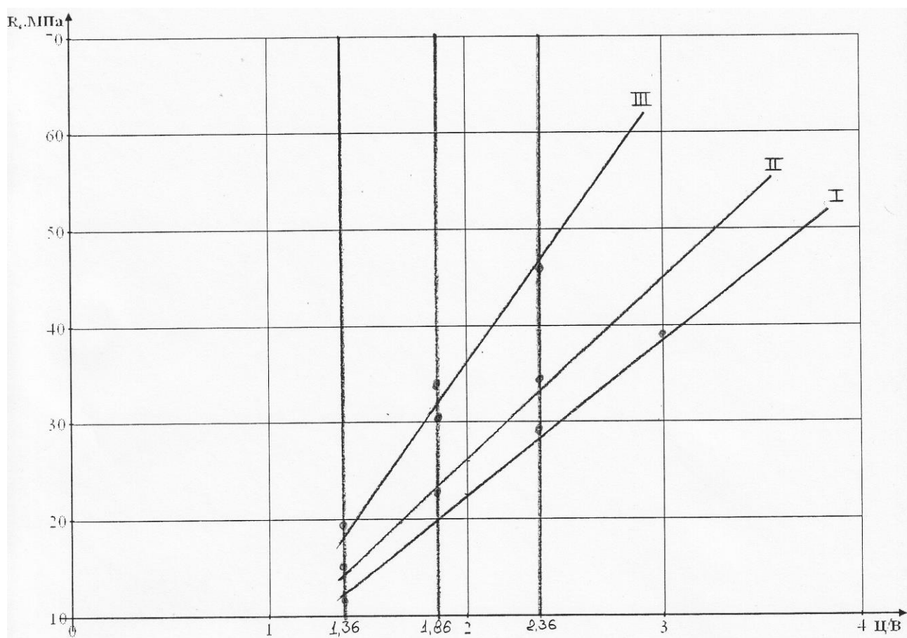
Рисунок 4.2 – Зависимость прочности бетона от цементно-водного отношения;
