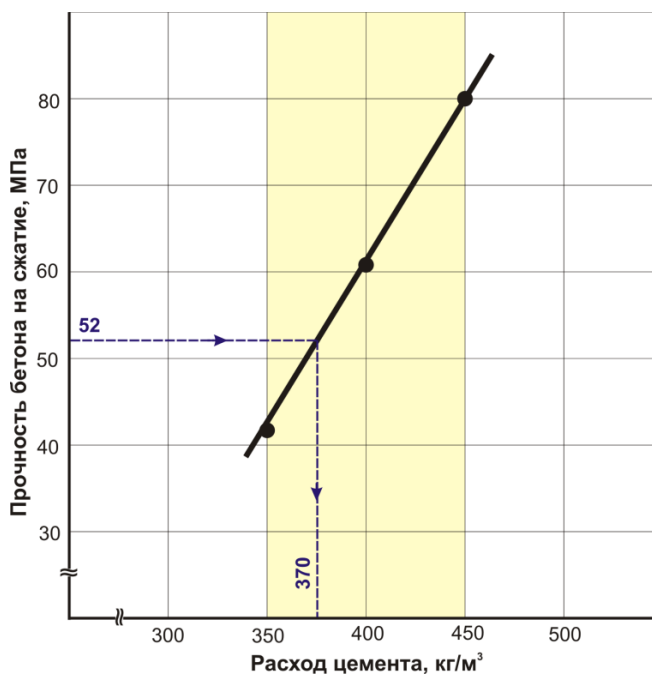
Рисунок 12.3 – Зависимость прочности бетона от расхода цемента
