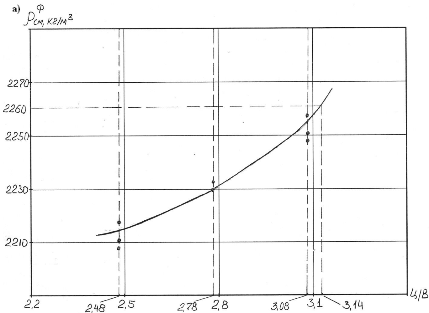
Рисунок 8.2 – Базовая зависимость «средняя плотность бетонной смеси – Ц/В-отношение»
