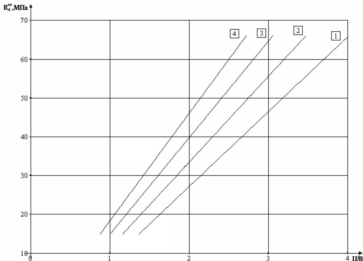
Рисунок 6.1 – Зависимость прочности мелкозернистого бетона через 28 суток нормального твердения от Ц/В отношения и класса прочности цемента; 1 –цемент ЦЕМ 22,5; 2 –цемент ЦЕМ 32,5; 3 – цемент ЦЕМ 42,5; 4 – цемент ЦЕМ 52,5
